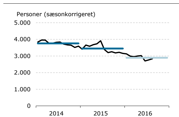
Figur 11 Registrerede arbejdssøgende
