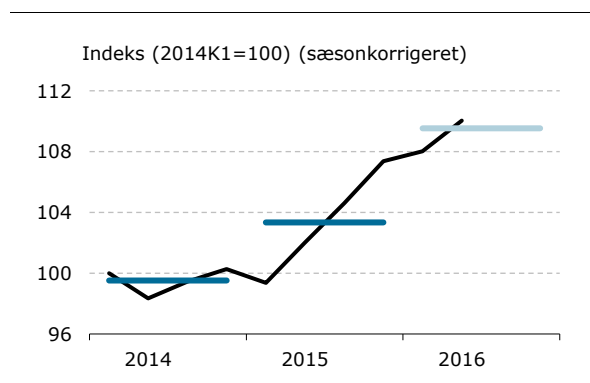
Figur 10 Detailomsætningen
