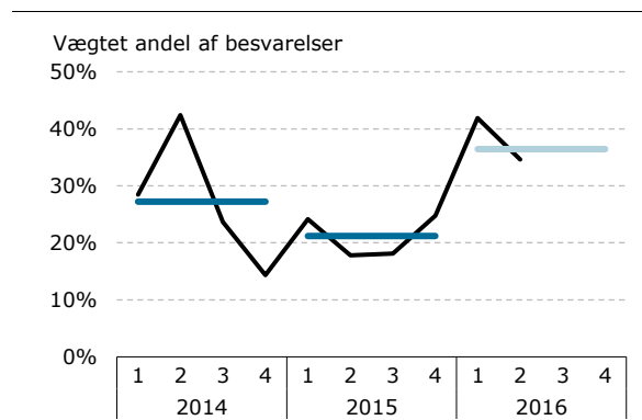
Figur 12 Virksomhedernes arbejdskraftmangel
