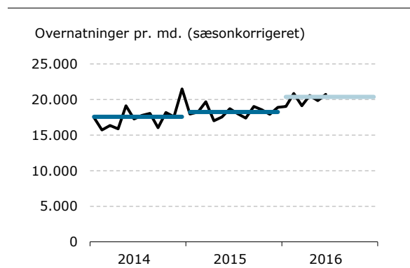
Figur 7 Hotelovernatninger
